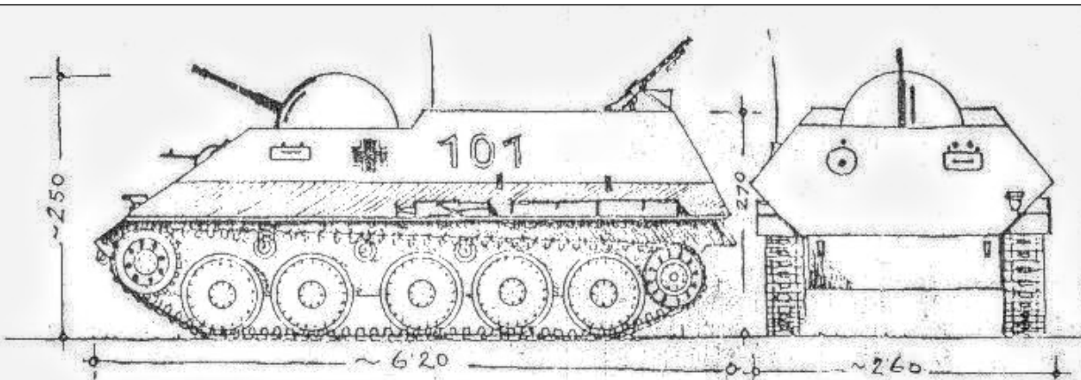
Deutscher Schützenpanzerwagen 1944
